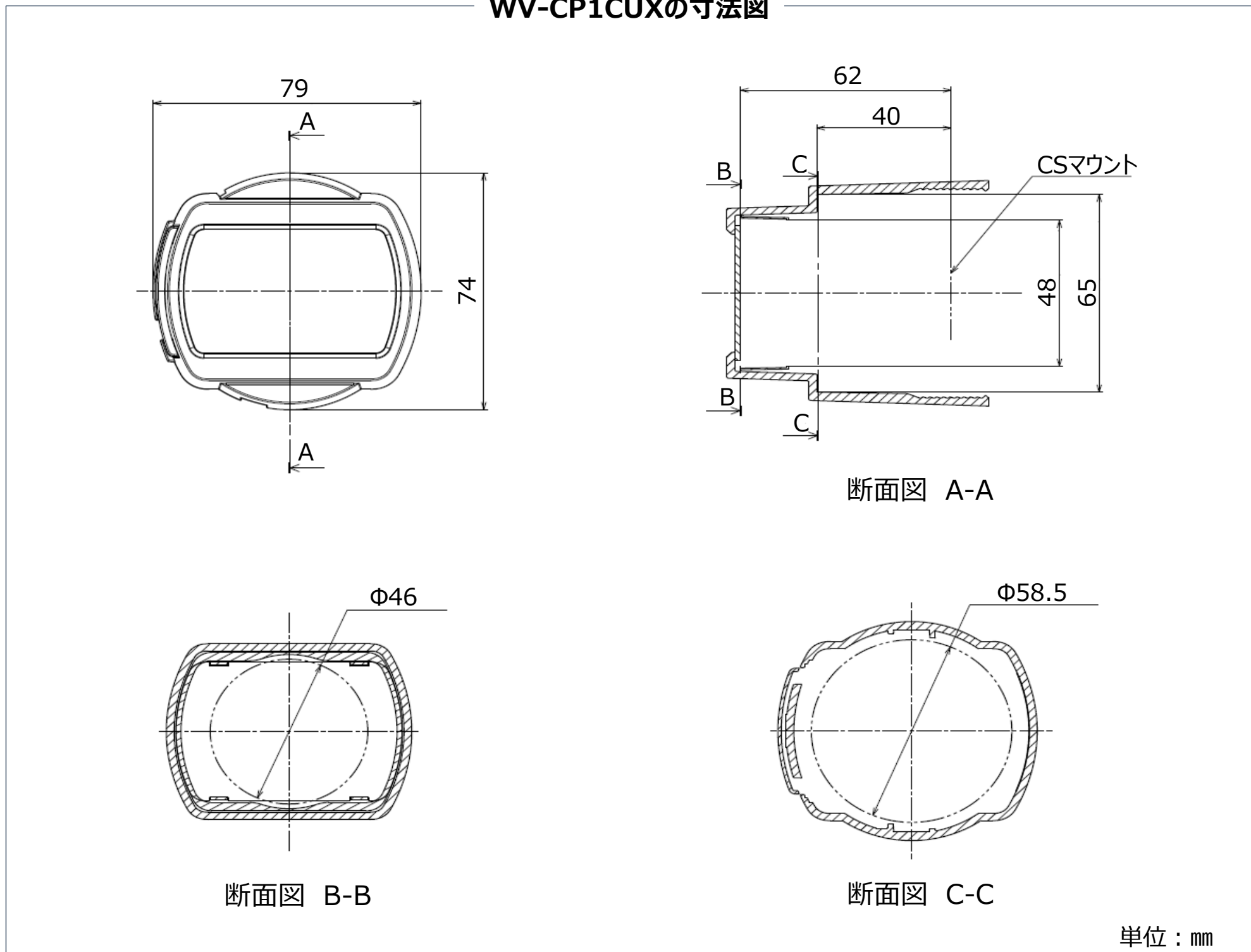
WV-CP1CUXの寸法図
