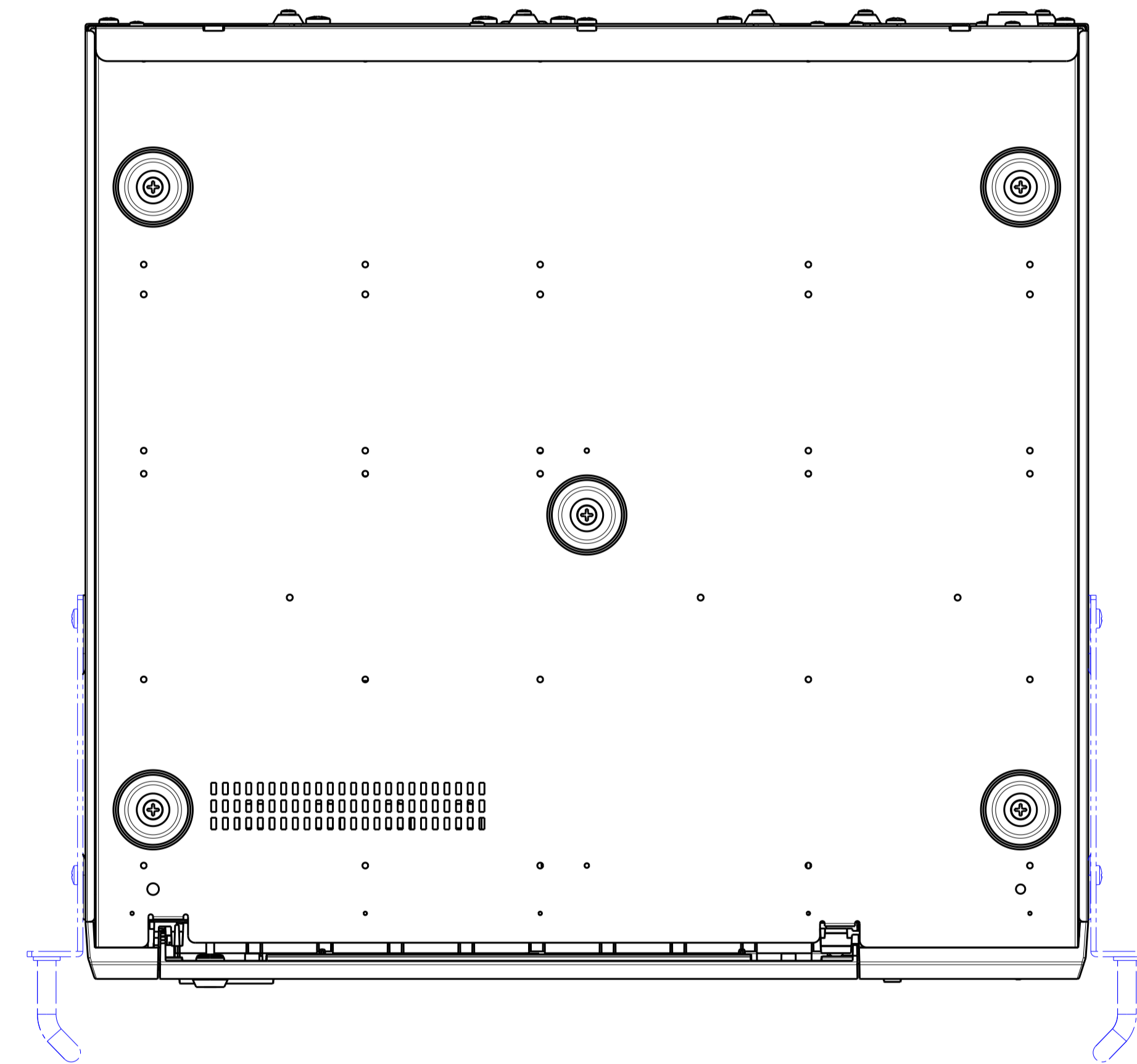
前面カバー開口状態 (HDDユニット装着時)
