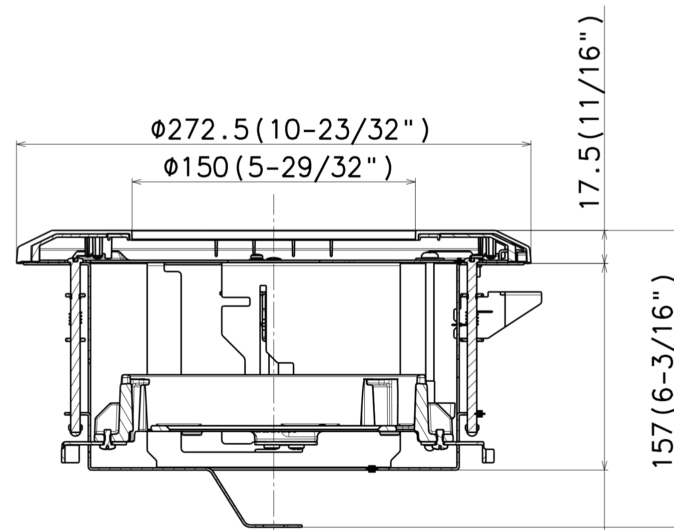
Sec A-A
