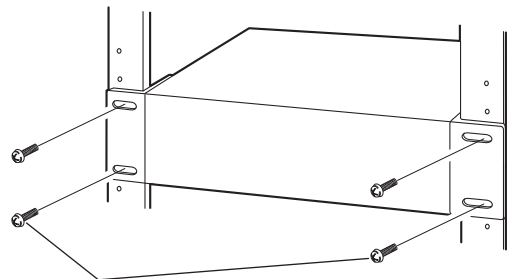
Vis de fixation d'équerre d'installation en bâti (M5 x 12, à se procurer localement)
