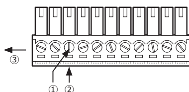
Fiche de raccordement (11 broches)
