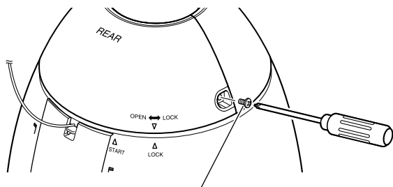
Parafuso de fixação do protetor solar anterior/ posterior
