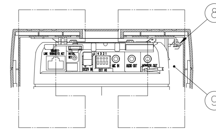
A-A 断面図
