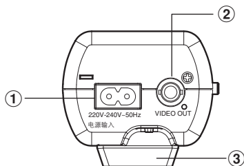
(后视图)
