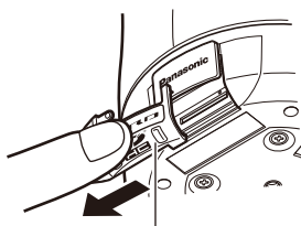
Cubierta de la ranura de la tarjeta de memoria SDHC/SD
