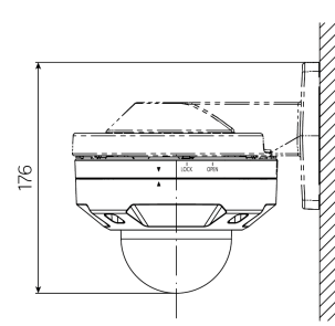
WV-QWL500** 組み合わせ例
