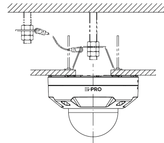
WV-Q105A** 組み合わせ例
