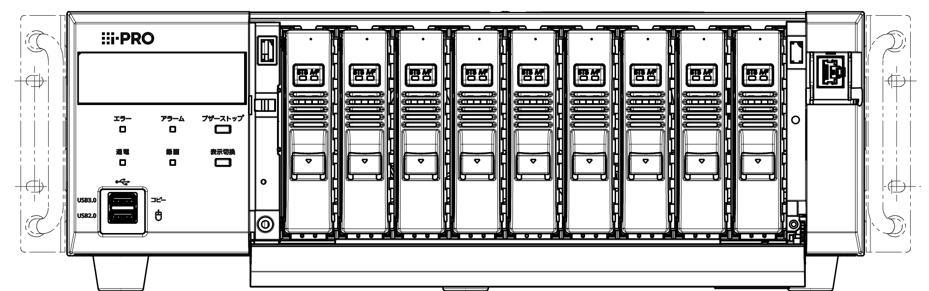
前面カバー開口状態
