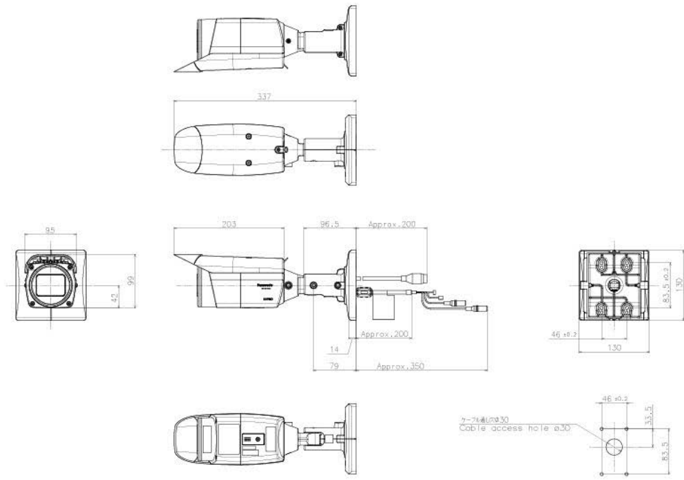
カメラ取り付け位置 Camera mounting position
