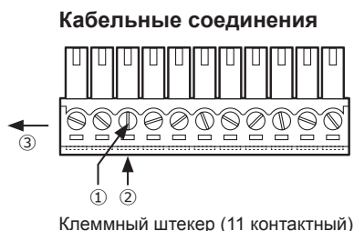
Гнезда разъемного соединителя сигнализации и контроля ALARM/CONTROL A
